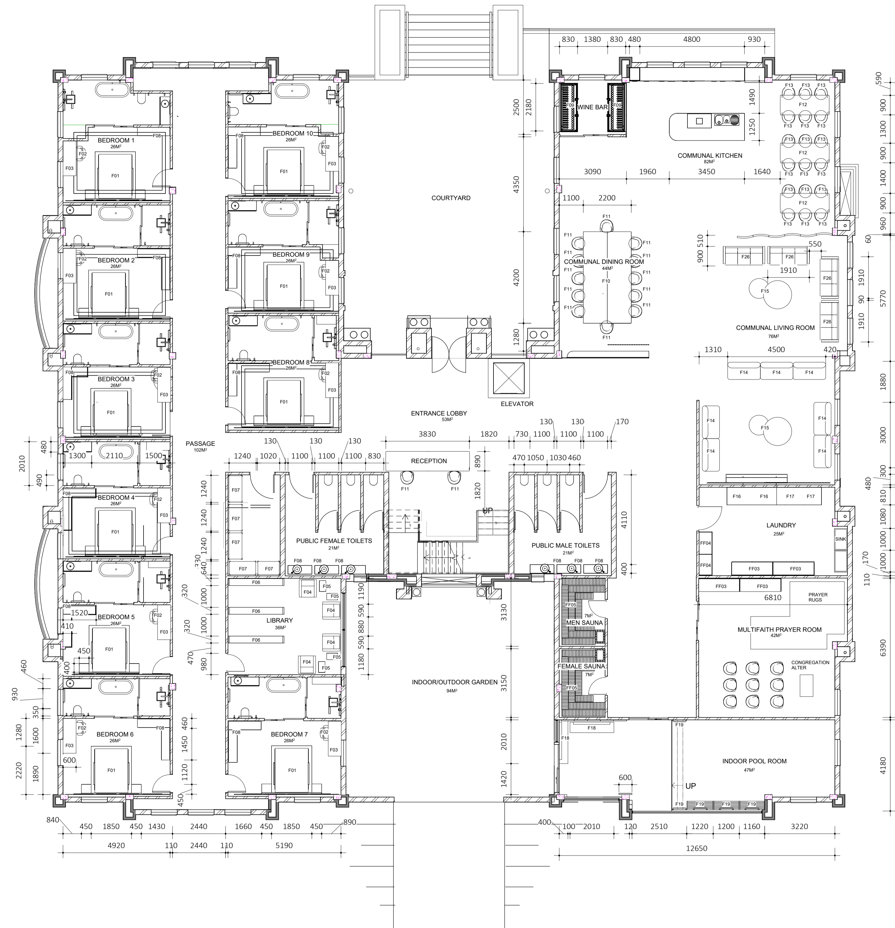
3.1 GF FF&E PLAN 1 : 100
