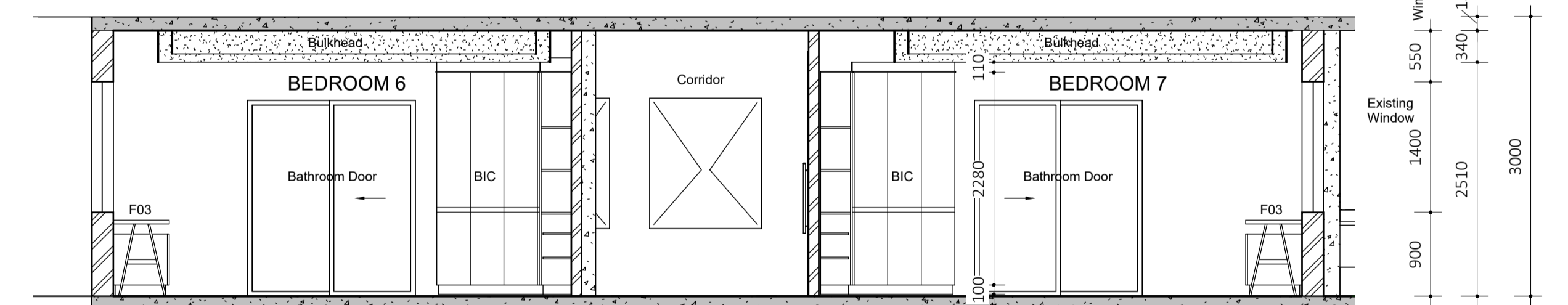
2.1 Section 1-1 1 : 50
