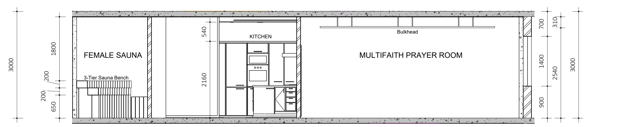
2.1 Section 3-3 1 : 50
