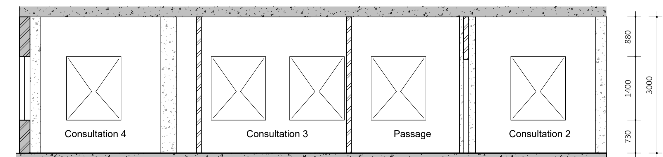
2.2 Section 4-4 1 : 50
