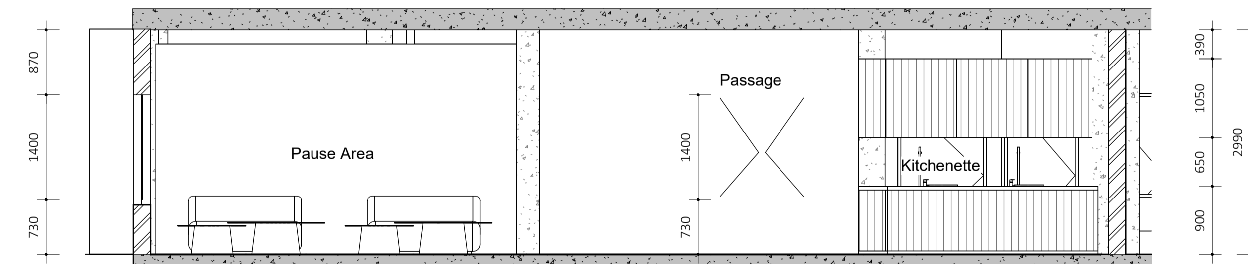
2.2 Section 2-2 1 : 50
